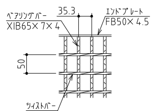
グレーチング構造図
